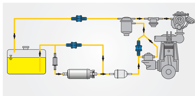
应用示例：带有切换式电动附加泵的化油器发动机
